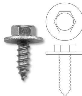
Tornillo Aleta 6,3 x 20mm Zincado (llave 10 SW) Cód. 0150.065.20
