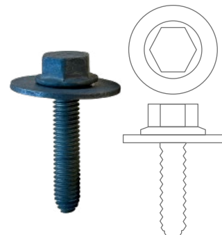
Tornillo hexagonal 6 x 30 con arandela 24 mm Cód. 0150.617.31
