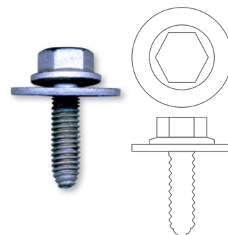
Tornillo 6 x 20 Renault Cód. 0900.617.24
