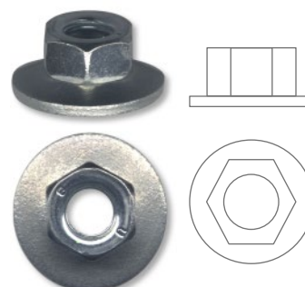
Tuerca con arandela móvil M8 BI Cód. 0150.458.13
