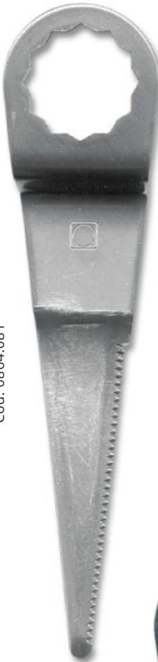
Recta dentada largo 85 corte 60 Cód. 0864.081
