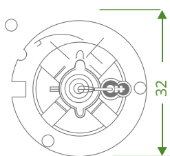
DESCARGA GAS XENÓN D2R 85V 35W Cód. 0085.074
