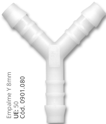
Empalme Y 6mm UE: 50 Cód. 0901.060
