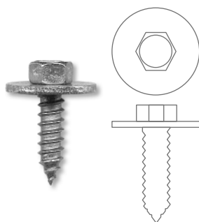
Tornillo Aleta 5,5 x 19mm zincado (llave 8 SW) Cód. 0150.055.19
