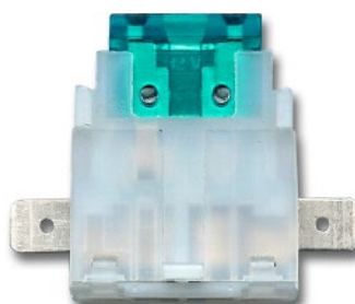
Aéreo Faston enchufe later Cód. 0025.004
